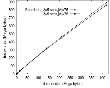
(d) TEC: 75 symbols
